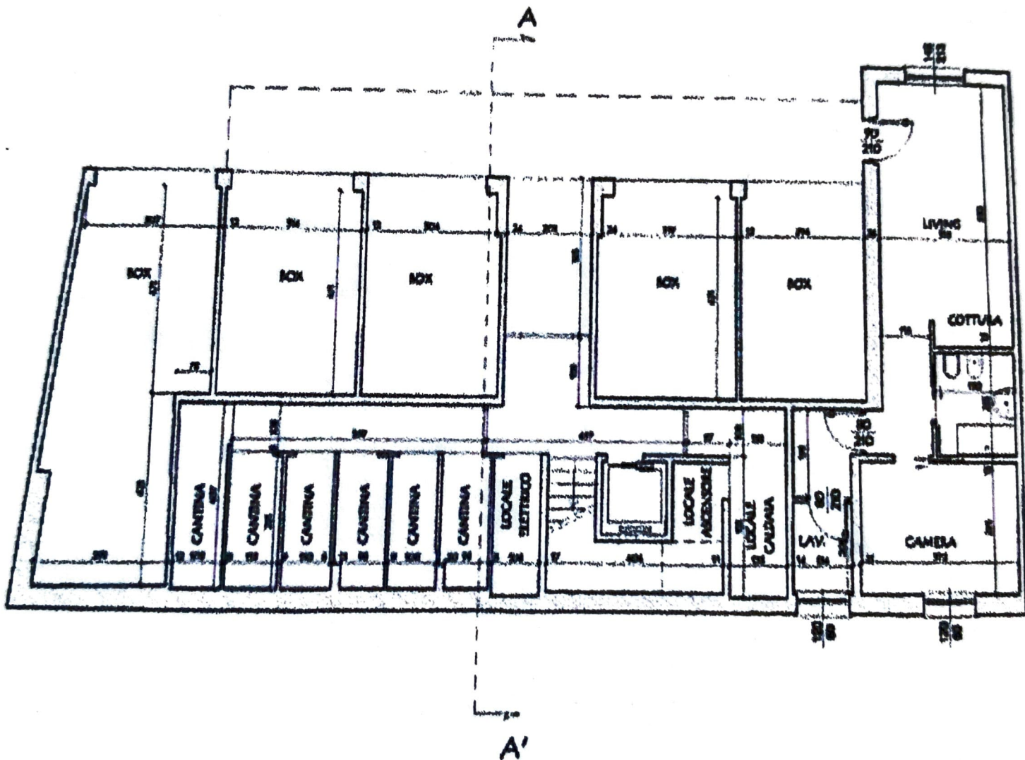
PIANTA PIANO TERRA STATO DI FATTO - SCALA 1:100
